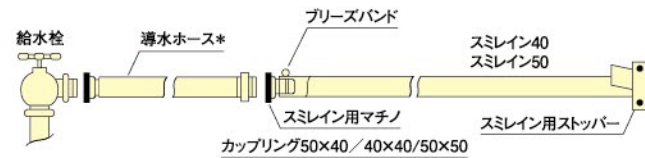
スミレイン専用継手を使用した敷設例
