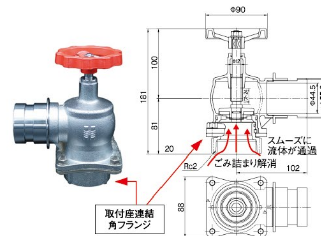
商品記号:SV-12N(BR) 90°
